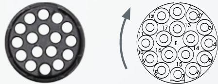
Ansicht steckseitig mating view
